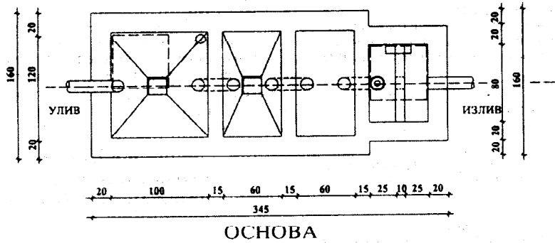
ТИП 1 - СЕПТИЧКА ЈАМА СА ТАЛОЖНИЦАМА И ДЕЗИНФЕКЦИЈОМ ПОМОЋУ ХЛОРИНАТОРА
