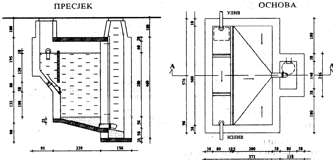
ТИП 2 - ЕМШЕРОВА ЈАМА ПРАВОУГАОНОГ ОБЛИКА М 1 : 100
